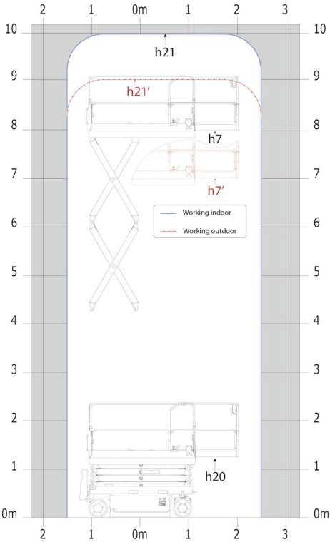
Lastdiagramm für Hubarbeitsbühne
