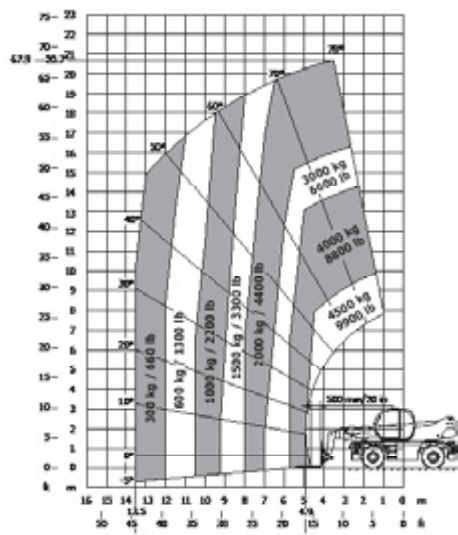
Rotierend bei ausgefahrenen Stützen mit Seilwinde 1.500 kg EN 1459
