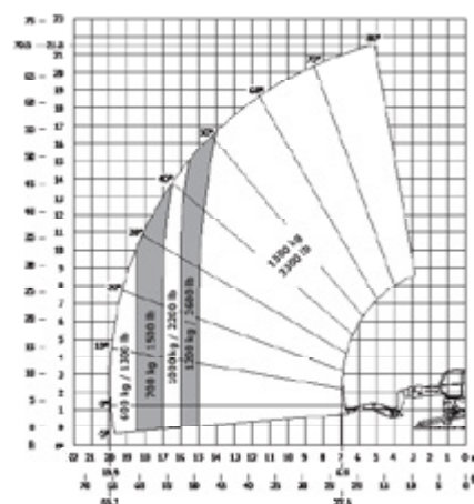
Rotierend bei ausgefahrenen Stützen mit Kranausleger 1.500 kg EN 1459
