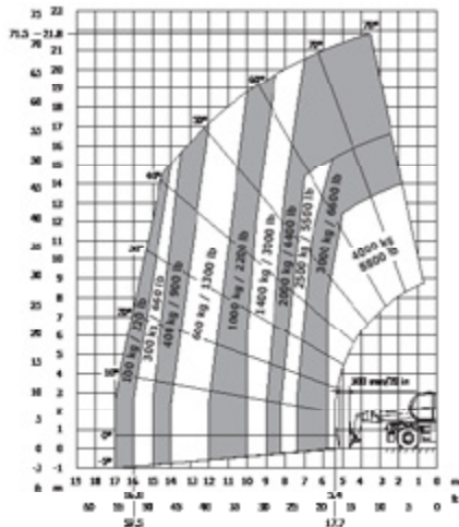
Frontal auf den Rädern mit Gabeln EN 1459
