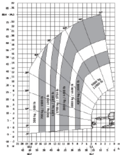
Rotierend bei ausgefahrenen Stützen Positive 3D-Arbeitsbühne EN 280
