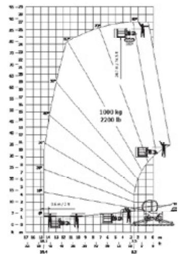
Rotierend bei ausgefahrenen Stützen mit Hubarbeitsbühne 1.000 kg EN 280
