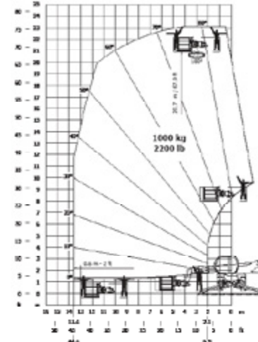
Rotierend bei ausgefahrenen Stützen mit Hubarbeitsbühne 1.000 kg EN 280
