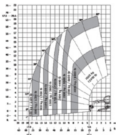
Rotierend bei ausgefahrenen Stützen Positive 3D-Arbeitsbühne EN 280
