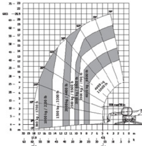
Rotierend bei ausgefahrenen Stützen mit Gabeln EN 1459
