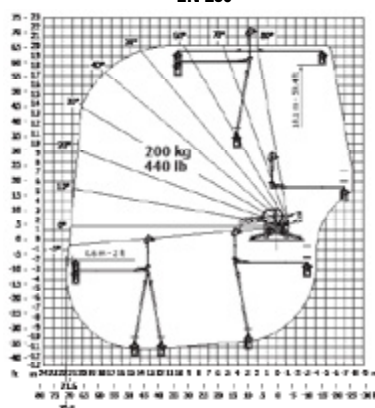
Rotierend bei ausgefahrenen Stützen Negative 3D-Arbeitsbühne EN 280
