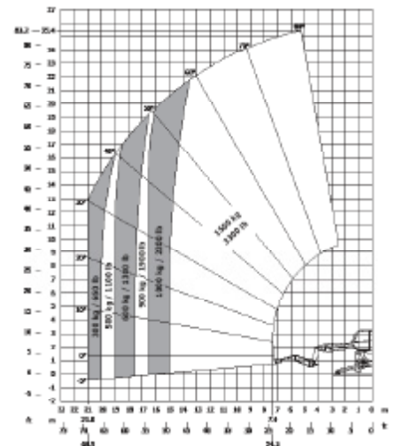
Rotierend bei ausgefahrenen Stützen mit Hubarbeitsbühne 1.000 kg EN 280
