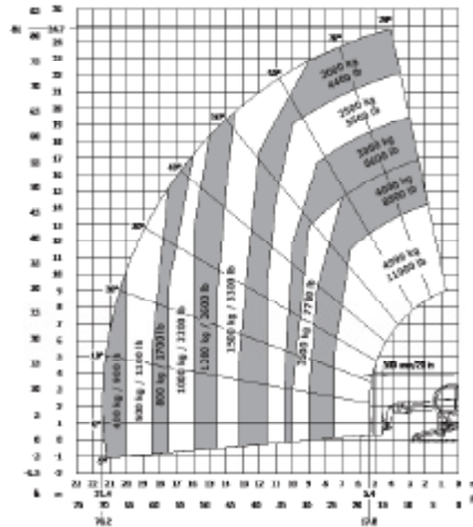
Rotierend bei ausgefahrenen Stützen mit Gabeln EN 1459
