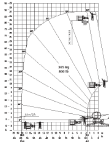
Rotierend bei ausgefahrenen Stützen mit Hubarbeitsbühne 365 kg EN 280
