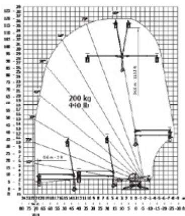
Rotierend bei ausgefahrenen Stützen Positive 3D-Arbeitsbühne EN 280
