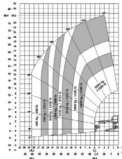
Rotierend bei ausgefahrenen Stützen mit Seilwinde 5.000 kg
