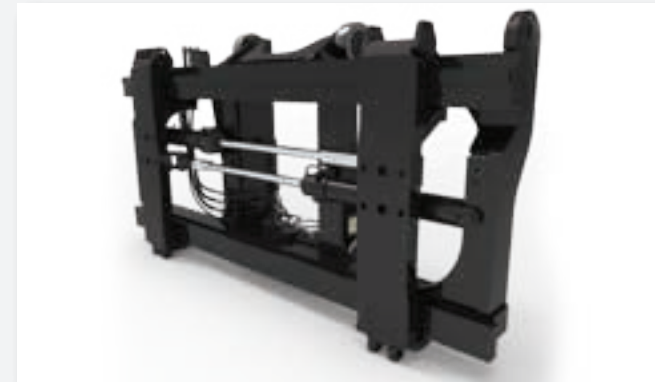
3.040 mm breiter Doppelfunktionsgabelträger mit Seitenschub und Gabelzinkenverstellung – einzeln verstellbare Gabelzinken – Gabelzinken mit Hakenaufhängung
