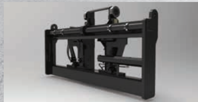
3.100 mm breiter Seitenschubrahmengabelträger – wellengeführte Gabelzinken
