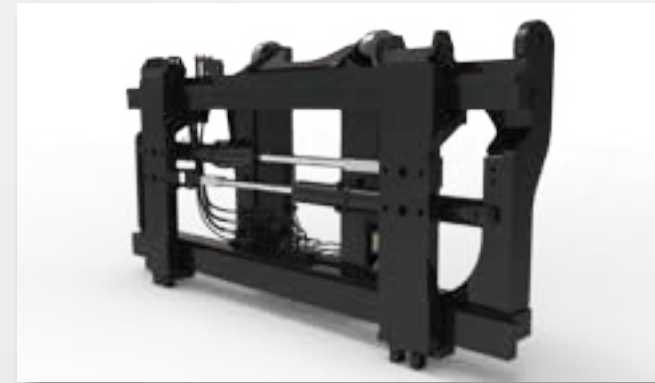
3.200 mm breiter Mehrzweck-Doppelfunktionsgabelträger mit Seitenschub und Gabelzinkenverstellung – einzeln verstellbare Gabelzinken – Gabelzinken mit Hakenaufhängung
